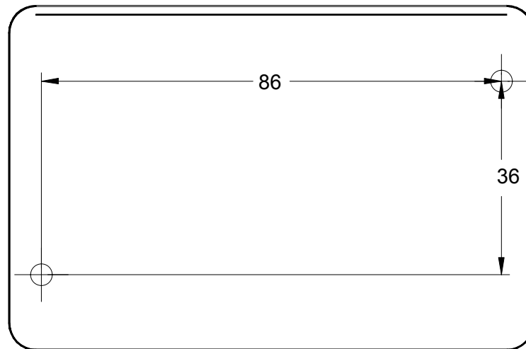
Bild 4 Standardgehäuse
